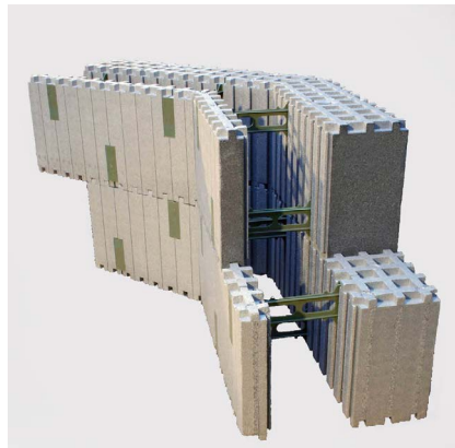
Eckstückelemente MCFU 35 „rechts“ und „links“.
