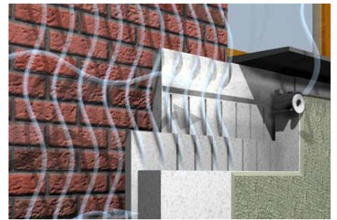
Montage der Platte IZOBETA
