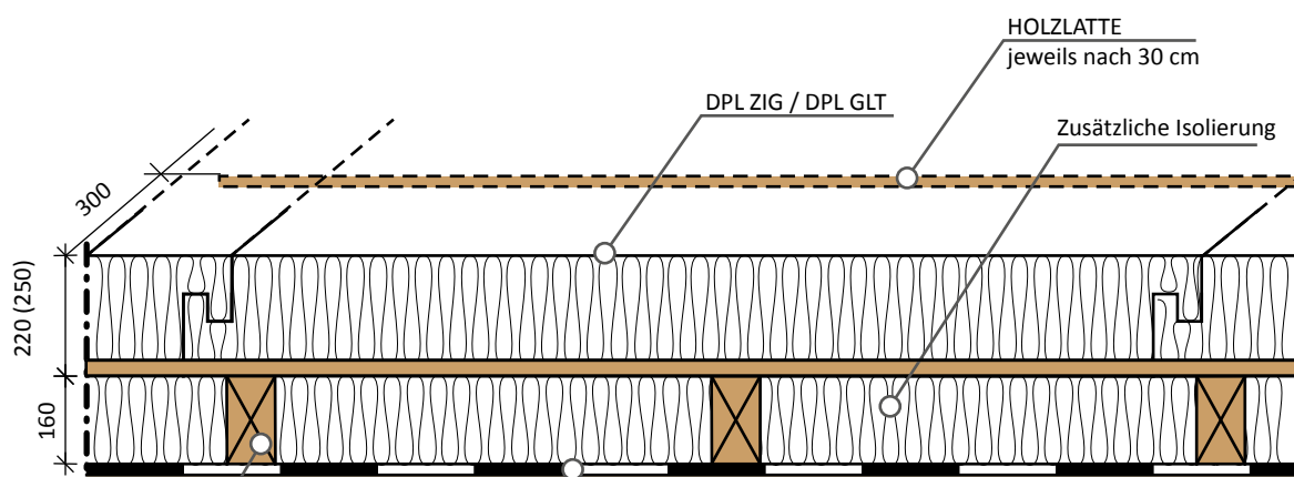
Rys. B Horizontaler Querschnitt durch eine Dachfläche mit zusätzlicher Isolierung zwischen den Sparren.
