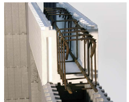
Im Sturzelement ML ist das Verlegen der Bewehrung einfach.
