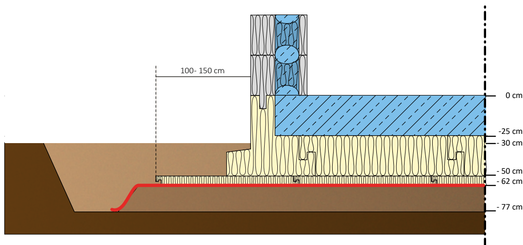
Abb. 2 Schema der Fertigung des Plattenfundaments mit der Anwendung einer zusätzlichen thermischen Isolierung.
