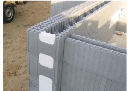
Baut man die Leibungen und stumpfe Wandabschlüsse – die Öffnungen in der Verschalung, schließt man mit den Elementen OH, OB und OC.
