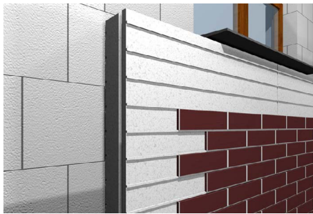
Funktionsschema der Platte IZOALFA
