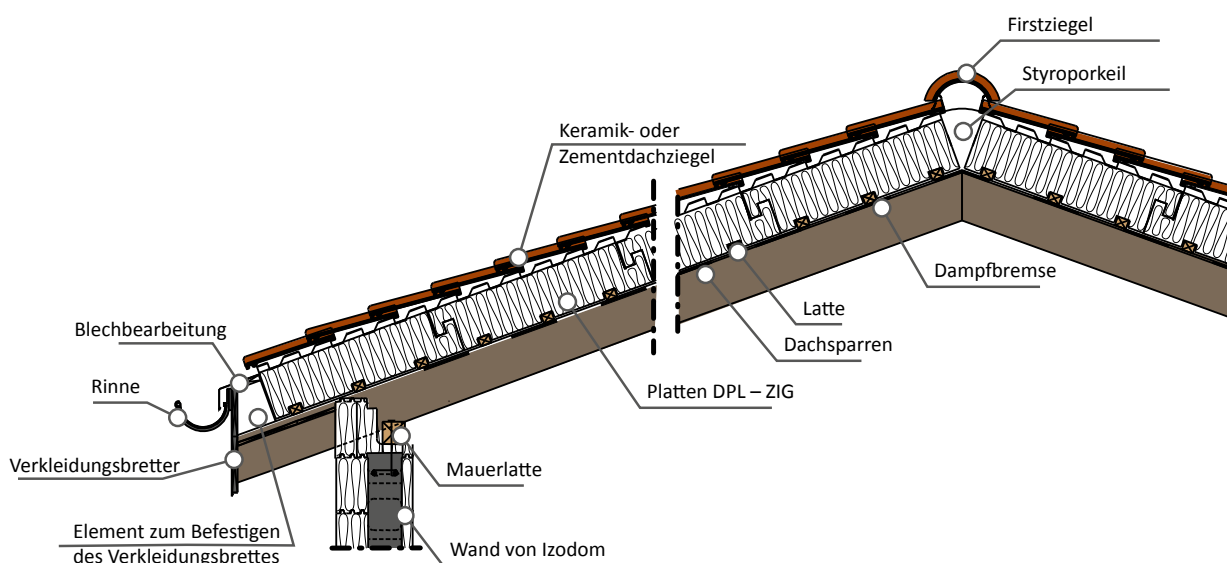
Rys. C Vertikaler Querschnitt, der die Variante der Dachbedeckung mit Dachziegeln - Biberschwanzziegeln illustriert.
