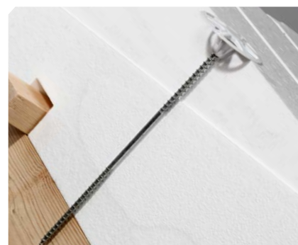
Spreizdübel für die Montage der Dachplatten von Izodom.
