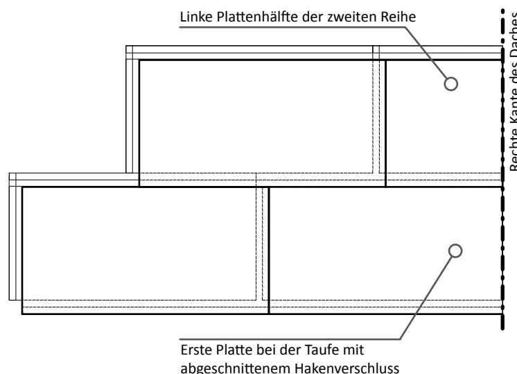
Rys. A Schema der Verlegung von Dachplatten.
