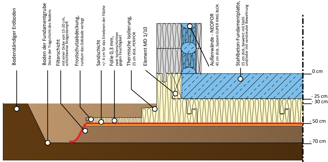
Abb. 1 Schema der Fertigung des Plattenfundaments in der Version mit den Außenwänden einer Breite von 45 cm (Super King Blok)
