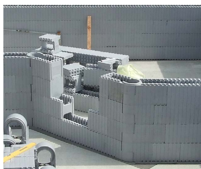
Anwendung von Scharnierelementen für die Gestaltung von Eckstücken unter einem beliebigen Winkel
