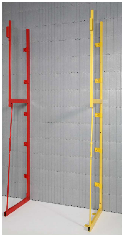
Die Stahlstützen erleichtern den Aufbau der Wand, die Kontrolle der Ebenen mit dem Erhalten des Vertikalen. Die Stützen mit roter Farbe sind für die Montage des Aufsatzes mit einer Höhe von 110 cm geeignet.
